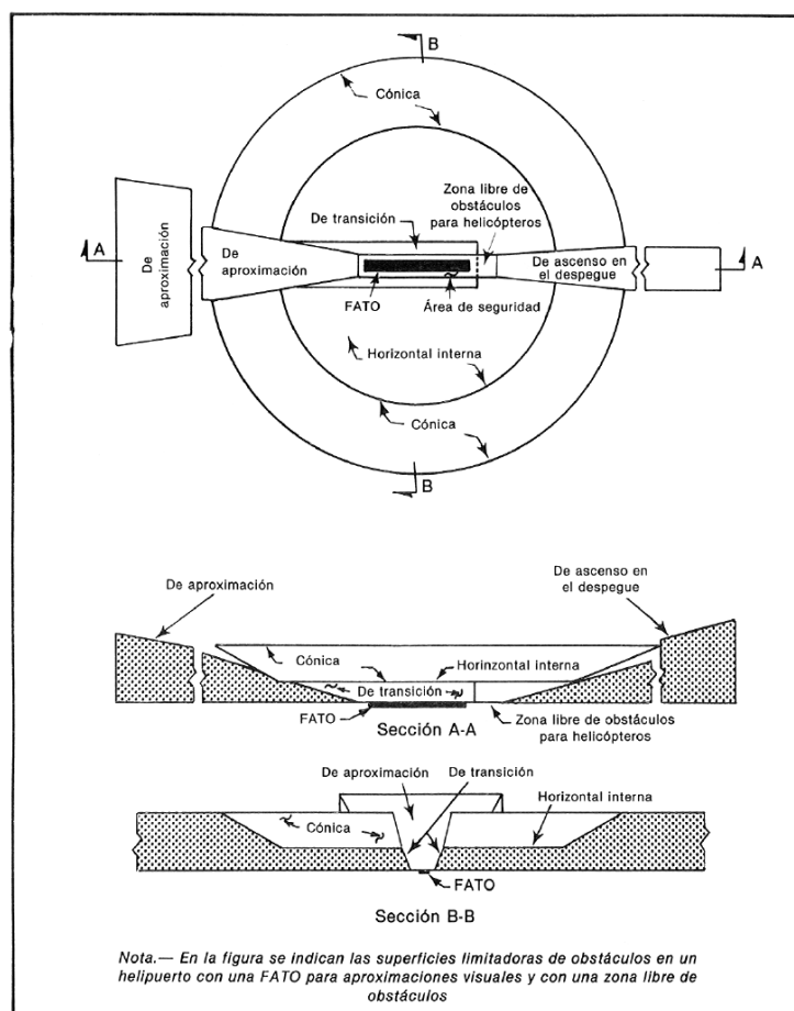
Figura 4-1H. Superficies limitadoras de obstáculos
