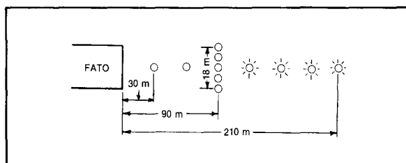
Figura 5-10H. Sistema de luces de aproximación
