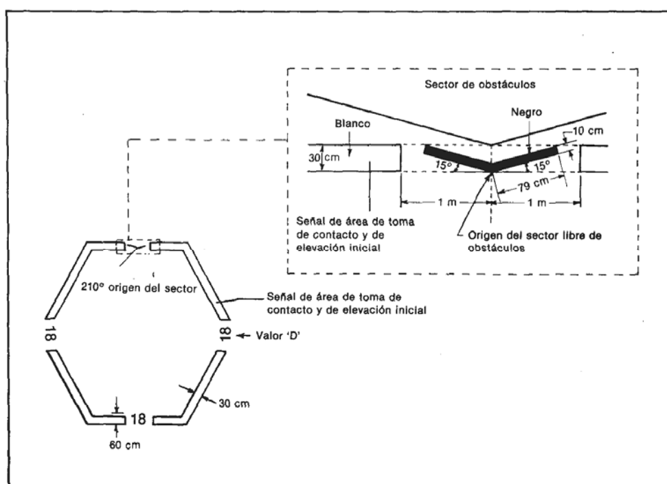
Figura 5-5H. Señal de sector despejado de obstáculos de heliplatforma
