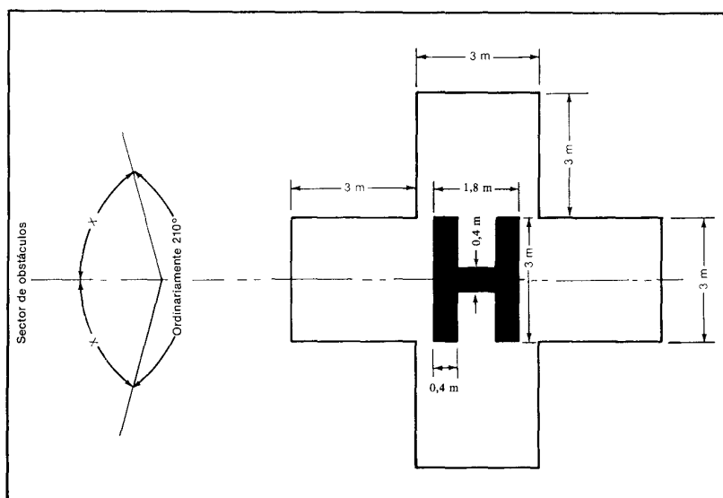
Figura 5-1H. Señal de identificación de helipuerto (indicada con una cruz de hospital y orientada con el sector despejado de obstáculos)
