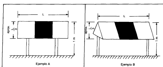
Figura 5-7H. Baliza de ruta de desplazamiento aéreo
