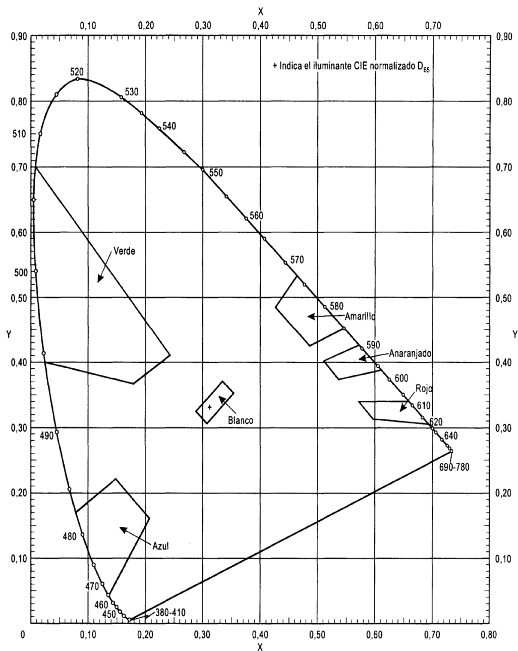
Figura A1 - 3. Colores de los materiales retroreflectantes para las señales, letreros y tableros
