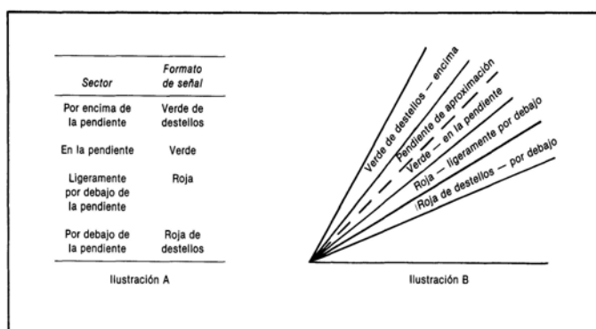
Figura 5-12H. Formato de la señal HAPI
