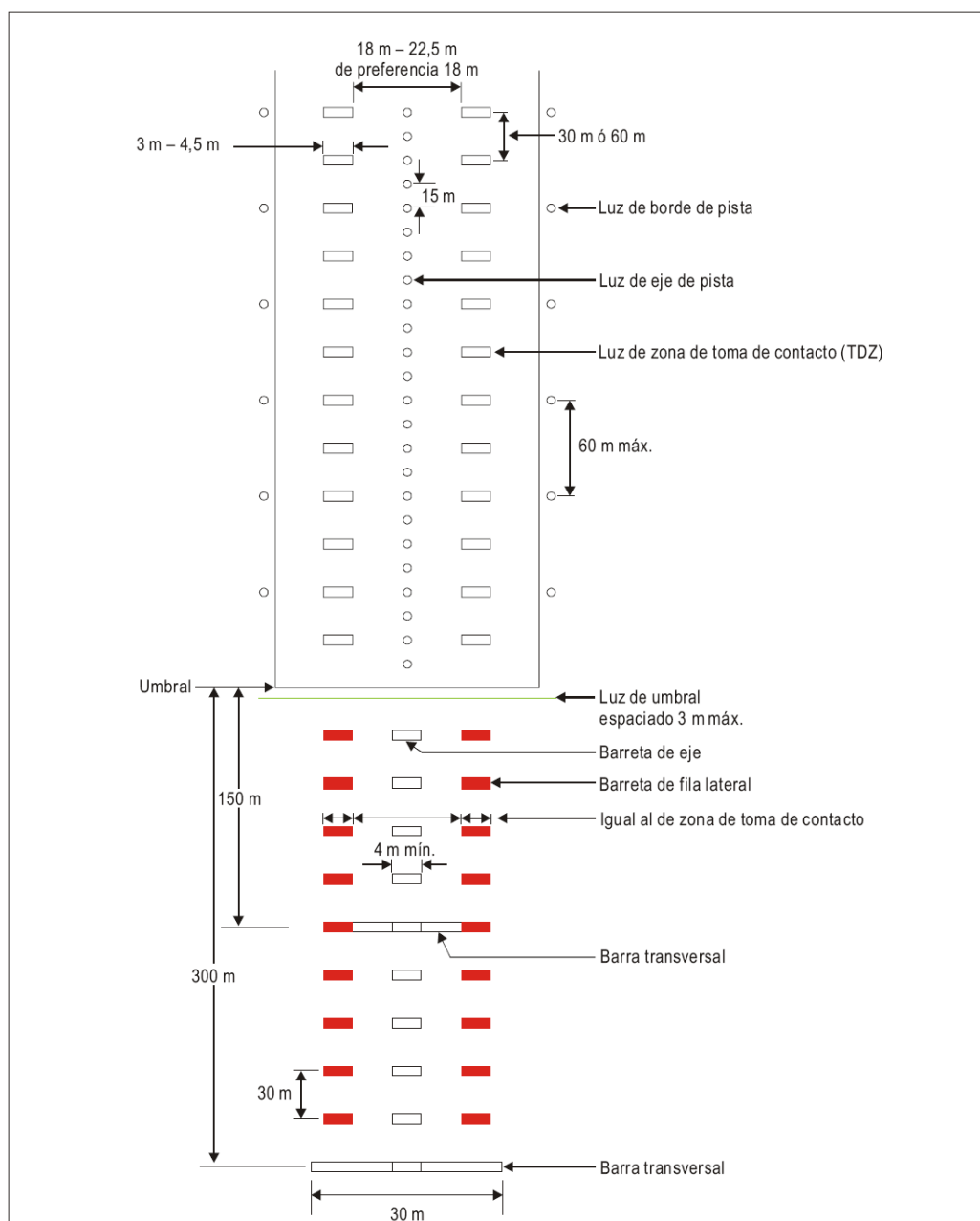
Figura 5-13. Iluminación de pista y de los 300m internos de la aproximación, en las pistas para aproximaciones de precisión de Categoría II y III
