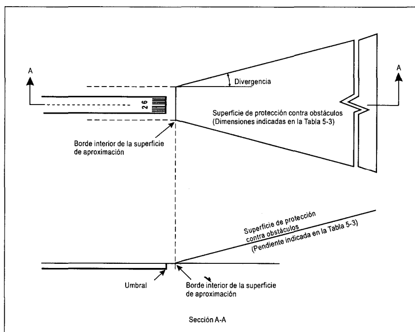
Figura 5-20. Superficies de protección contra obstáculos para los sistemas visuales indicadores de pendiente de aproximación
